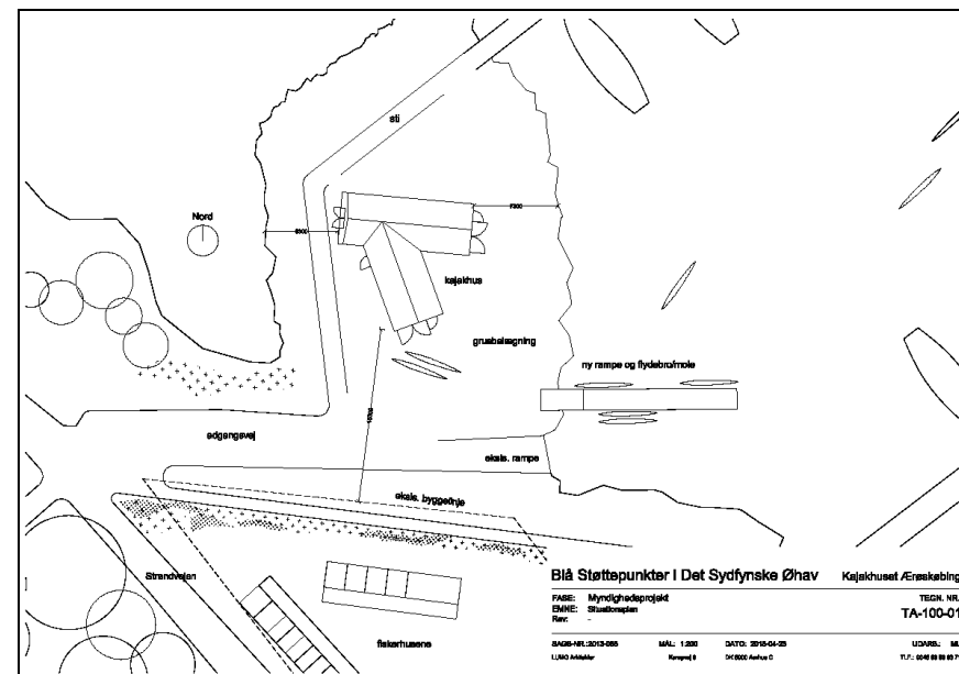
Tegninger af kajakhus og beliggenhed
